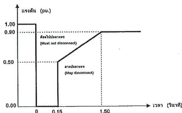
กราฟแสดงความสามารถในการทนต่อสภาวะแรงดันตกชั่วขณะ (Low voltage fault Ride through)
