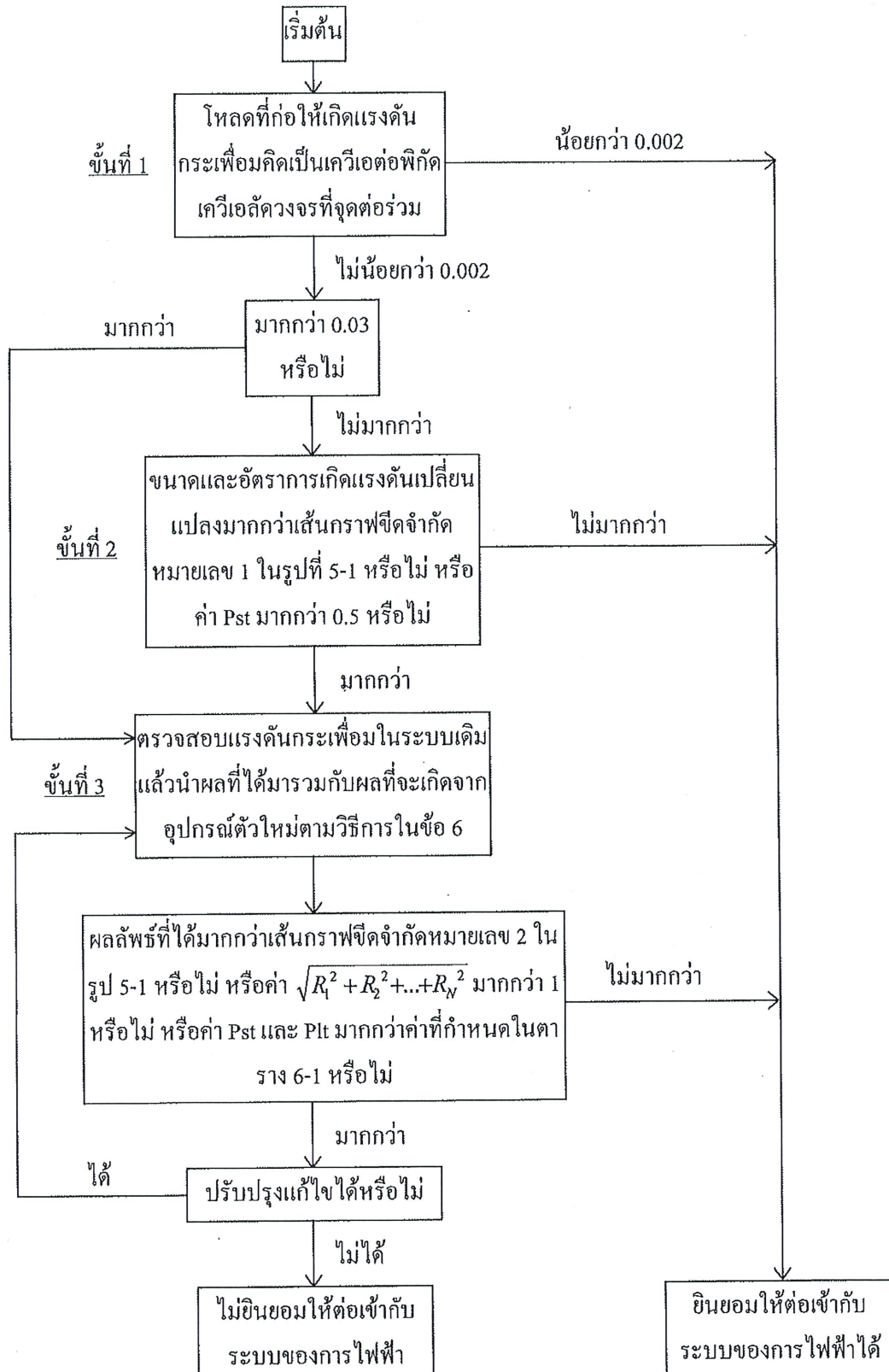
รูปที่ ผ-1 แผนผังลำดับขั้นตอนการตรวจสอบโหนดที่ก่อให้เกิดแรงดันกระเพื่อม
