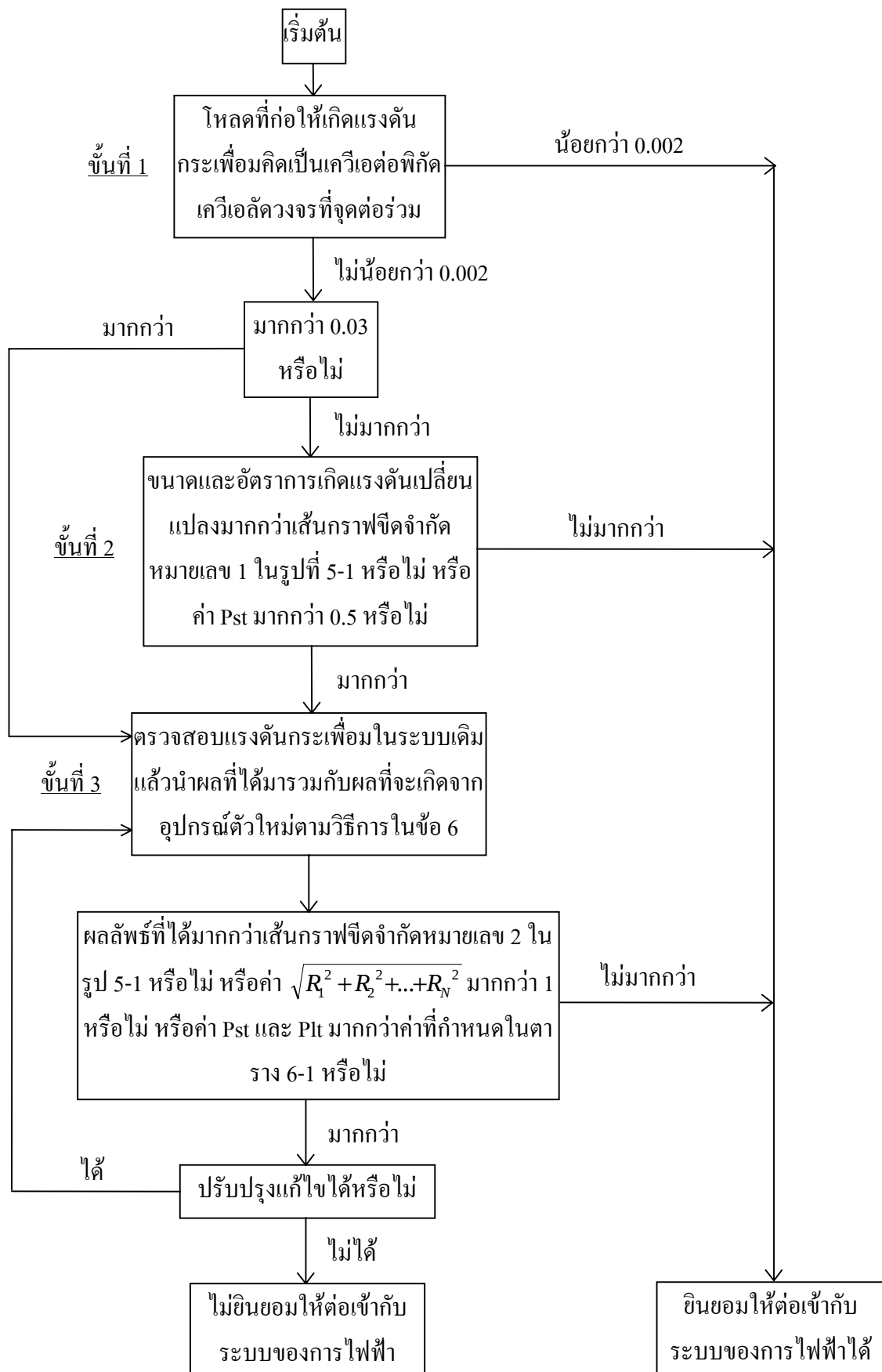
รูปที่ ผ-1 แผนผังลำดับขั้นตอนการตรวจสอบโพลต์ที่ก่อให้เกิดแรงดันกระพือ
