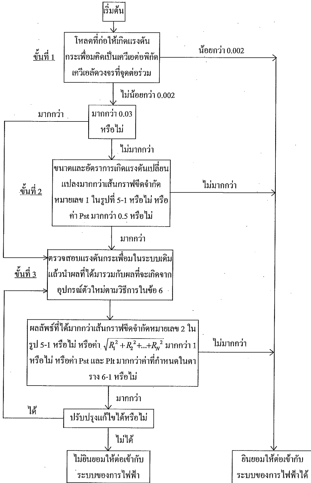
รูปที่ ผ-1 แผนผังลำดับขั้นตอนการตรวจสอบโหลดที่ก่อให้เกิดแรงดันกระแสเพิ่ม
